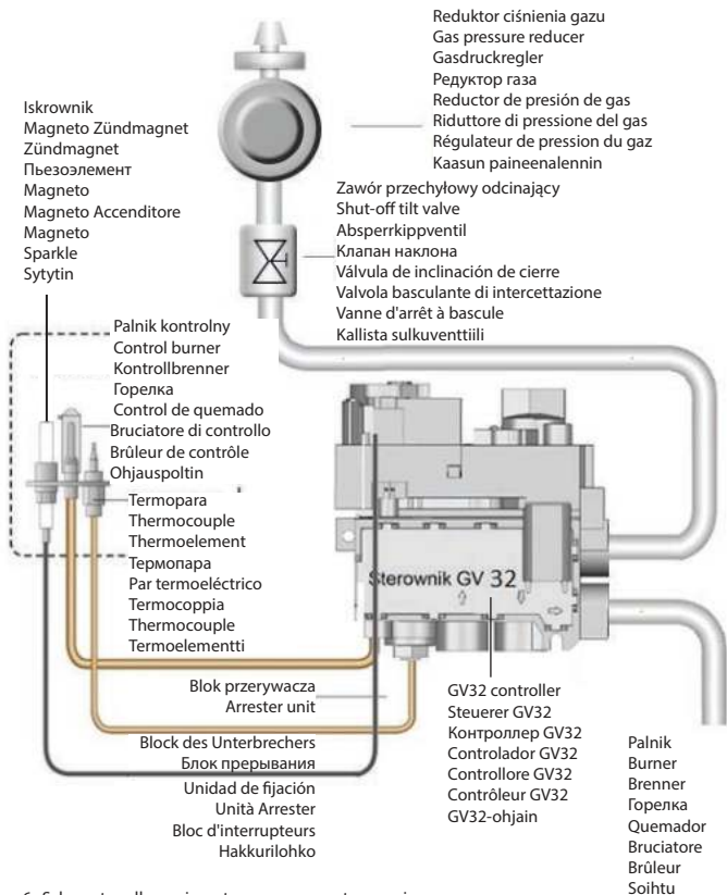
Rys. 6. Schemat podłączenia systemu ręcznego sterowania gazem
