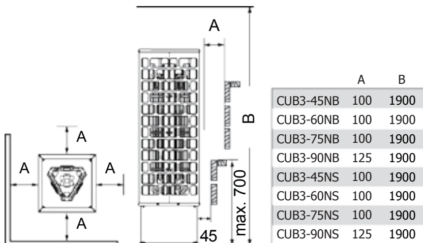
Kuva 2 | Minimisuojaetäisyydet (mm) Fig. 2 | Minimum safety distances (mm)
