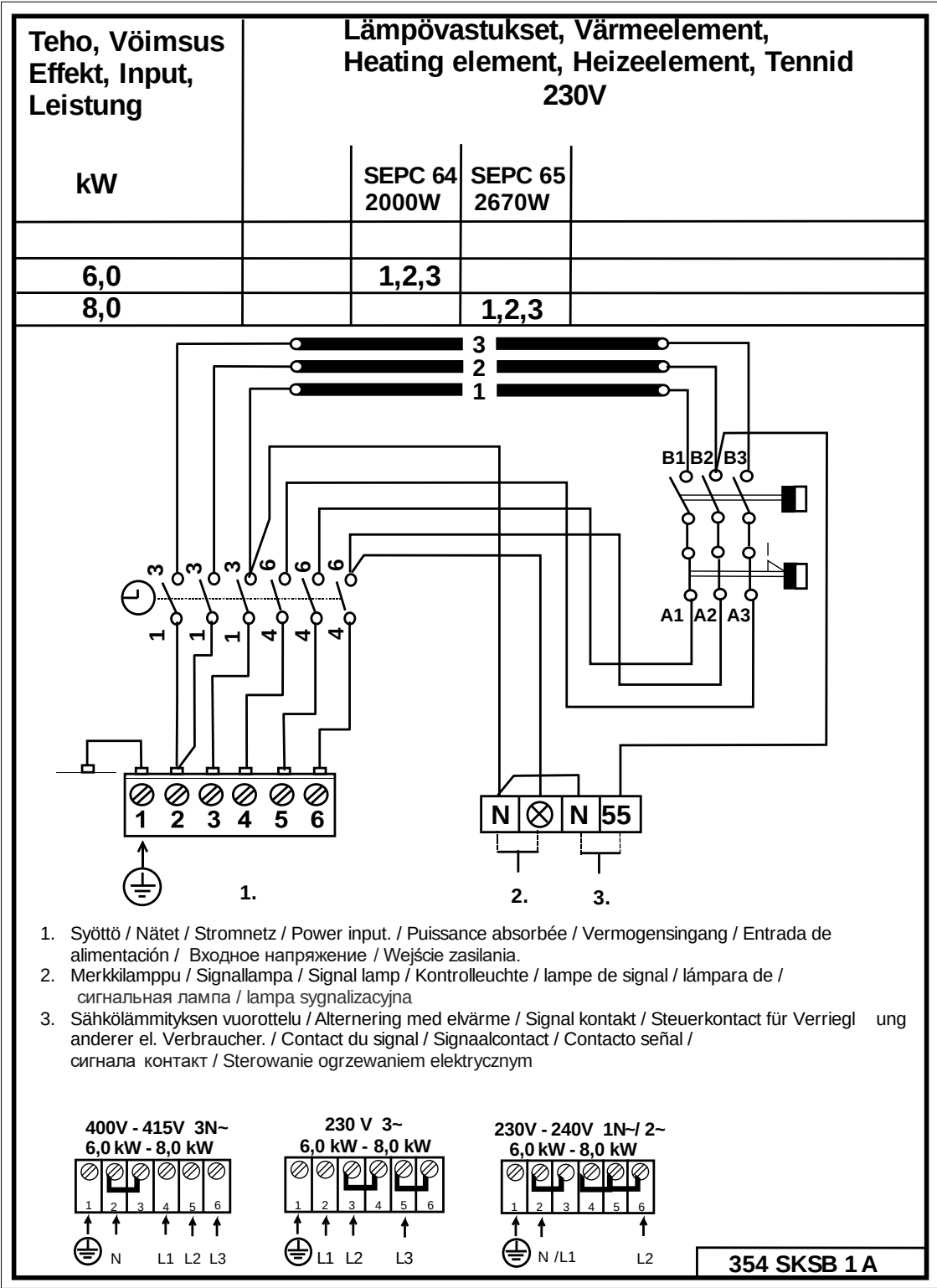
Abbildung 4 Schaltdiagramm
