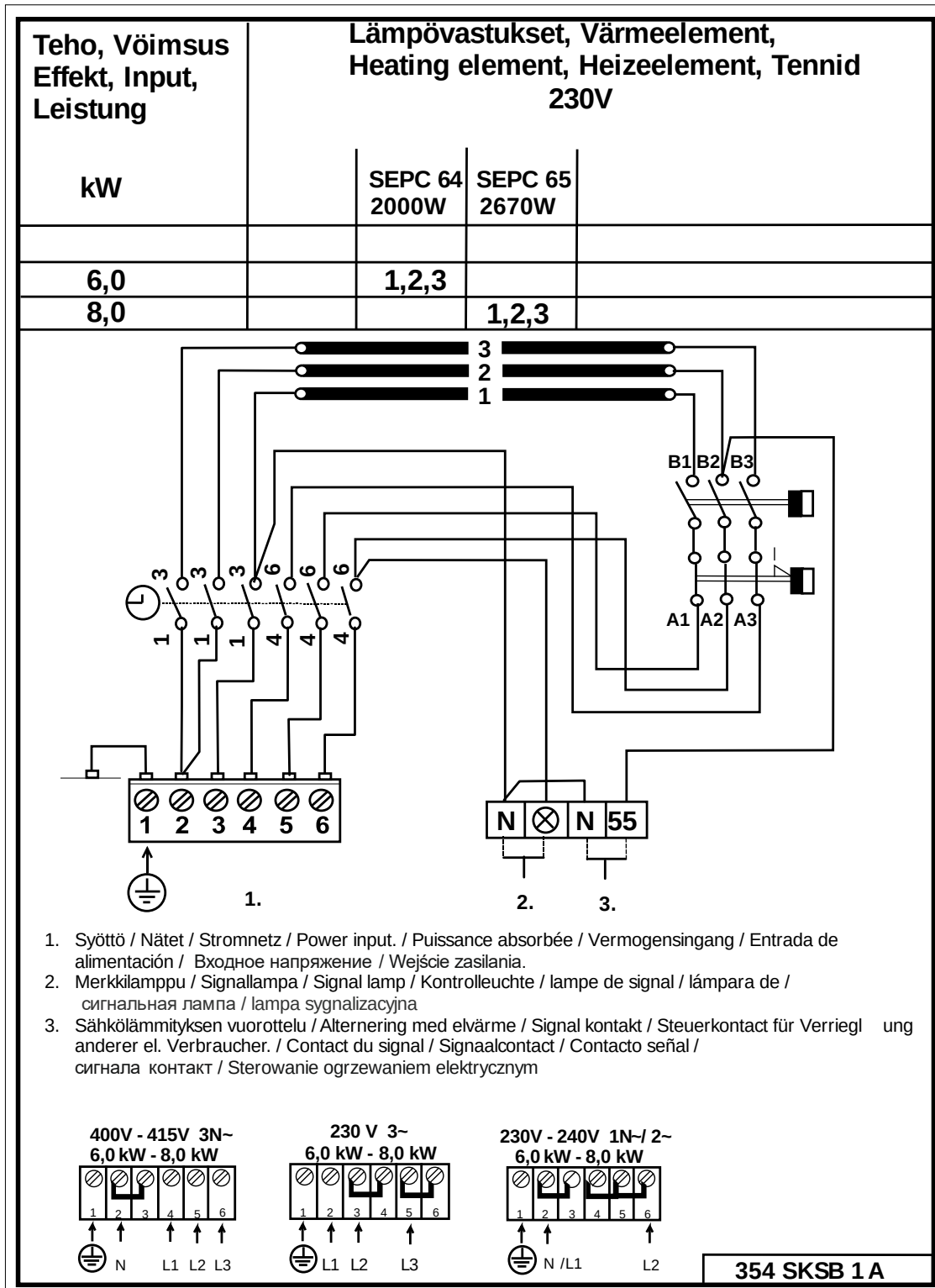
Kuva 4 KytKentäkaava
