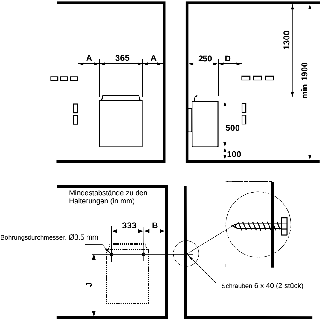
Abbildung 2 Sicherheitsabstände
