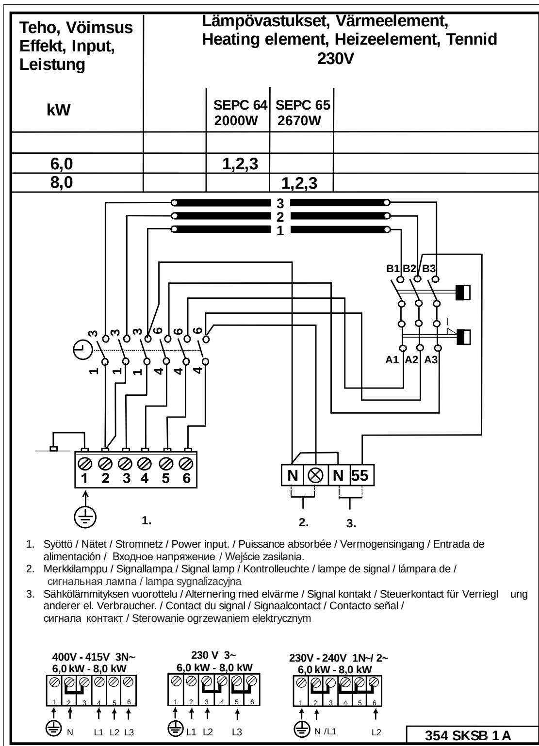
Bild 4 Kopplingsschema
