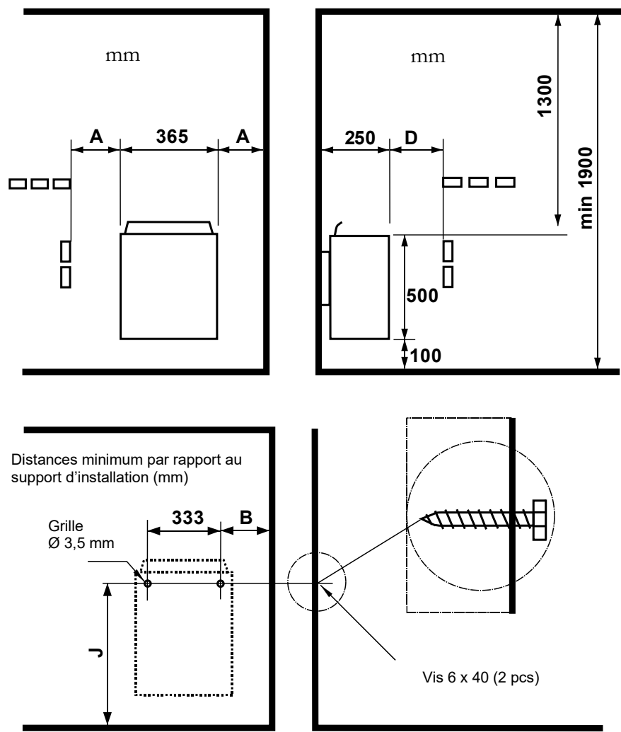
Illustration 2 Dégagements de sécurité
