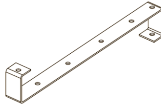
Osa 1, Kattokiinnike (korkeus kattopinnasta 70mm)
