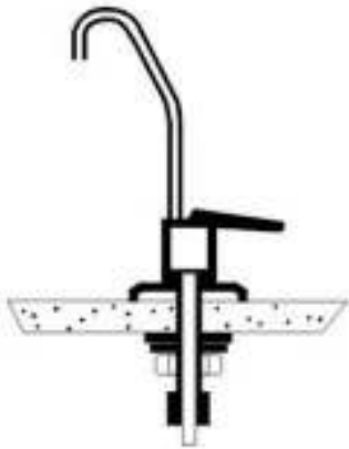
KUVA10. Hanan asennus työtasoon
