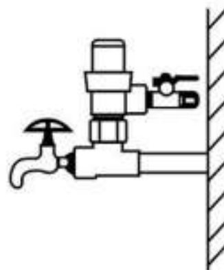
FIGUR 9. Tryckreduktionsventil
