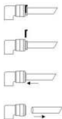
FIGUR 12. Lossa snabbanslutningen från PE-slangen
