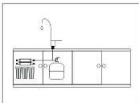
KUVA4. Asennus allaskaispistoon
