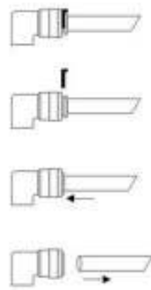
KUVA12. Pikaliitoksen irrotus PE-putkesta
