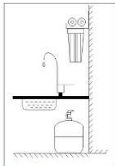
KUVA5. Asennus seinälle
