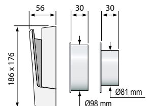
TL C Vaihtoventtiili
