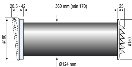
TL 80DE dBs Venttiili äv-kanavalla
