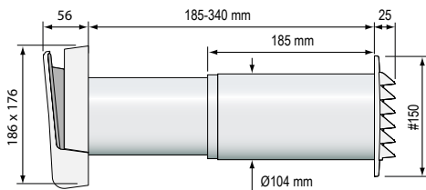
TL 100C Venttiilipaketti
