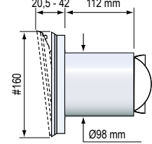
TL DE Vaihtoventtiili
