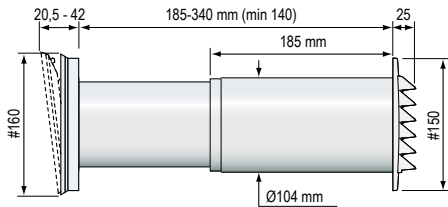
TL 100DE Venttiilipaketti
