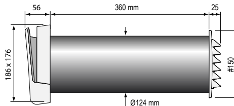
TL 80C dBs Venttiili äv-kanavalla
